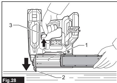
► 1. Magasin 2. Élément de contact 3. Gâchette
